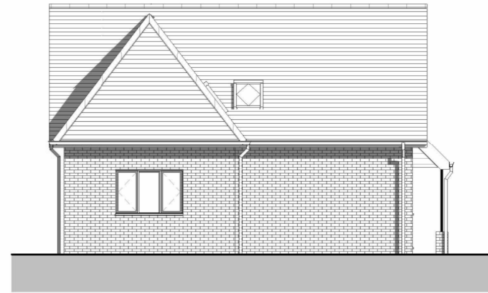
North 1 : 100
